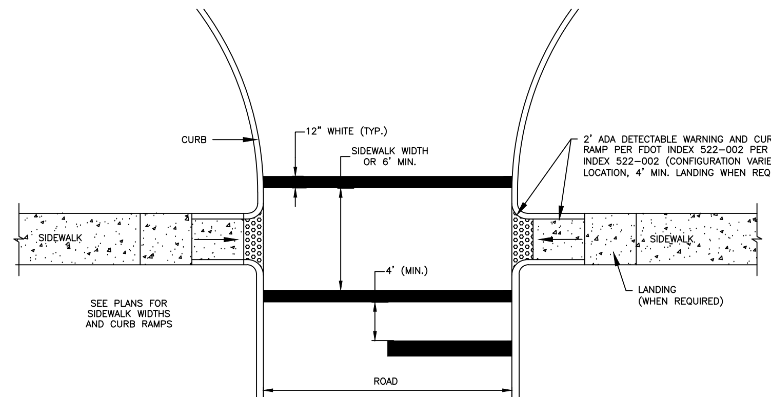
CROSSWALK DETAIL PER FDOT INDEX 711-001 N.T.S.
