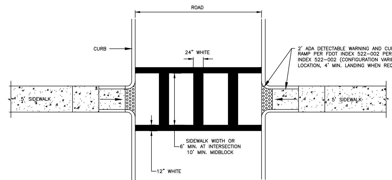
SPECIAL EMPHASIS CROSSWALK DETAIL PER FDOT INDEX 711-001 N.T.S.
